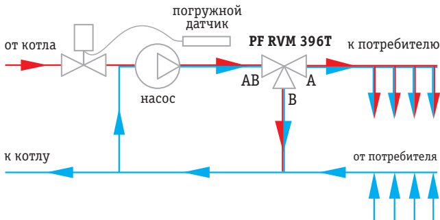
Схема 3. Регулирующий клапан PF RVM 396T на байпасе.
